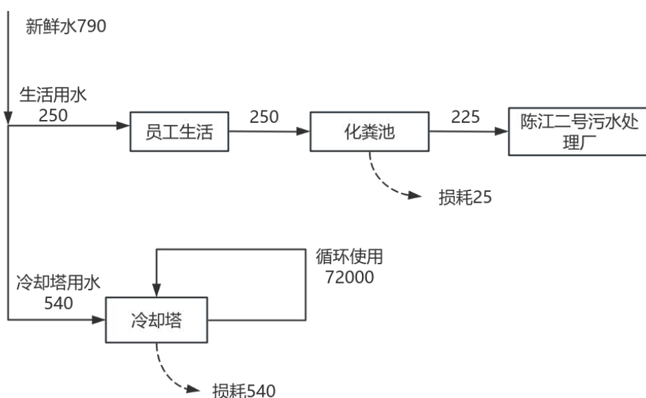
图 3-5 水平衡图 (t/a)
