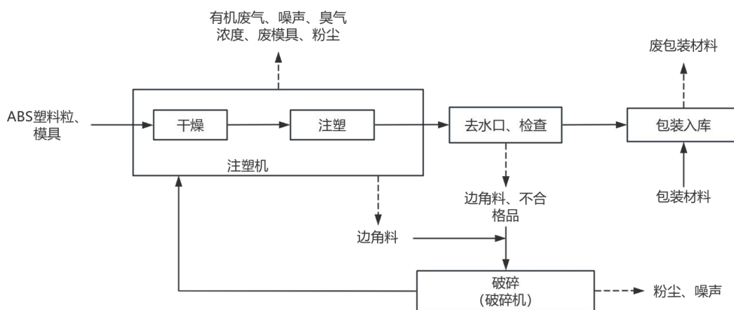
图 3-6 汽车塑料配件工艺流程及产污环节图
